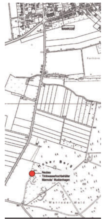
Der neue Behälter entsteht am Hohen Berg – neben dem alten Behälter.
