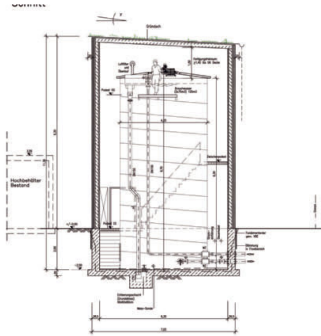
Etwa 11,5 Meter hoch wird das Bauwerk, in dem die zwei Trinkwasserbehälter stehen. Etwa zwei Meter tief wird das Gebäude in der Erde stehen. Skizzen: Ingenieurbüro Volmer
